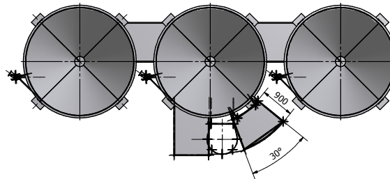
B-B ( 1:50 )
