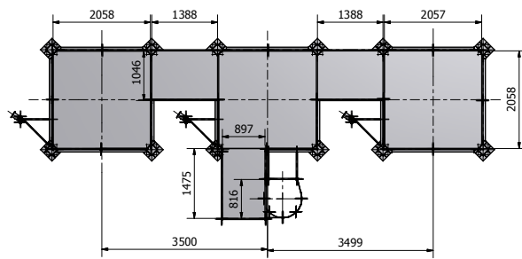
A-A ( 1:50 )
