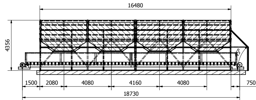
B-B ( 1 : 100 )
