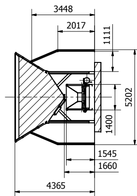
B-B ( 1 : 100 )
