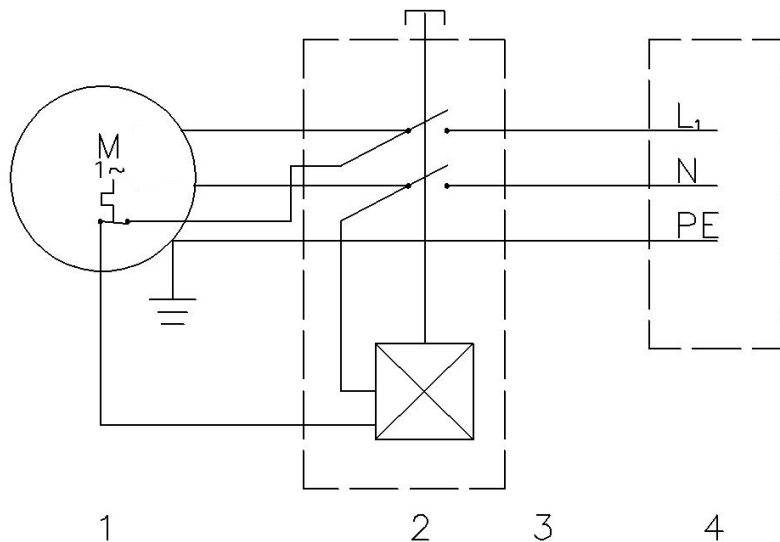
Rys. 2 Schemat elektryczny betoniarki POWER TEC 200L/230V/K
