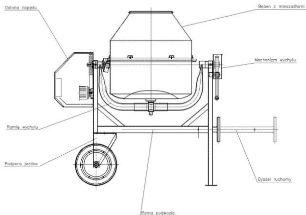
Rys. 1 Betoniarka elektryczna wolnospadowa POWER TEC 200L/230V/K (napęd wywrotu na korbę)
