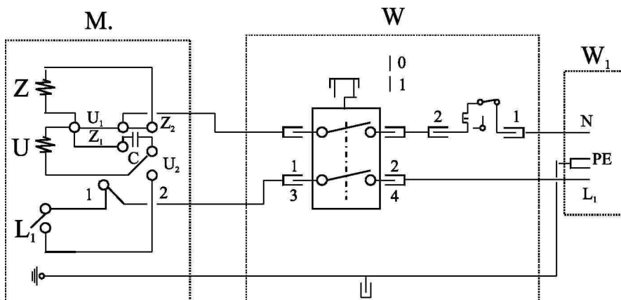
RYS NR 3. Schemat elektryczny betoniarki POWER TEC 280L/230V/O
