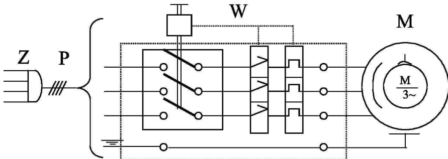
RYS NR 2. Schemat elektryczny betoniarki POWER TEC 280L/400V/O
